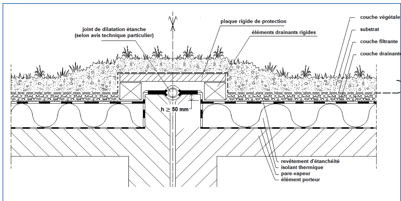
FIGURE 15 JOINT DE DILATATION RECOUVERT DE VÉGÉTALISATION
