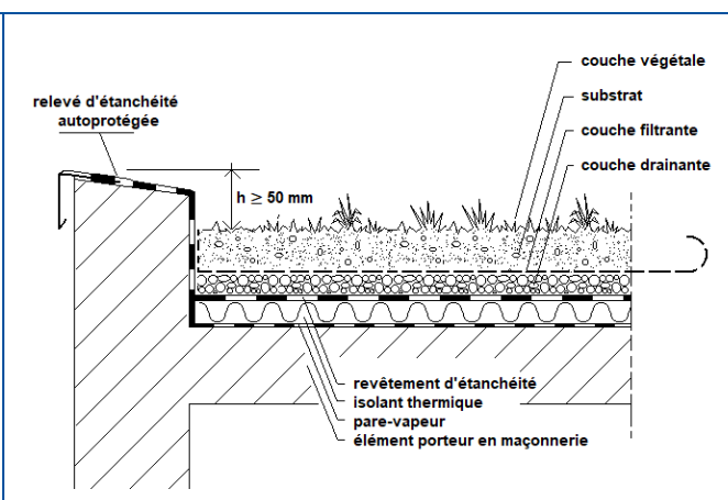
FIGURE 9 CAS OÙ L'ÉTANCHÉITÉ REVÊT L'ACROTÈRE : HAUTEUR DE RELEVÉ EN L'ABSENCE DE ZONE STÉRILE
