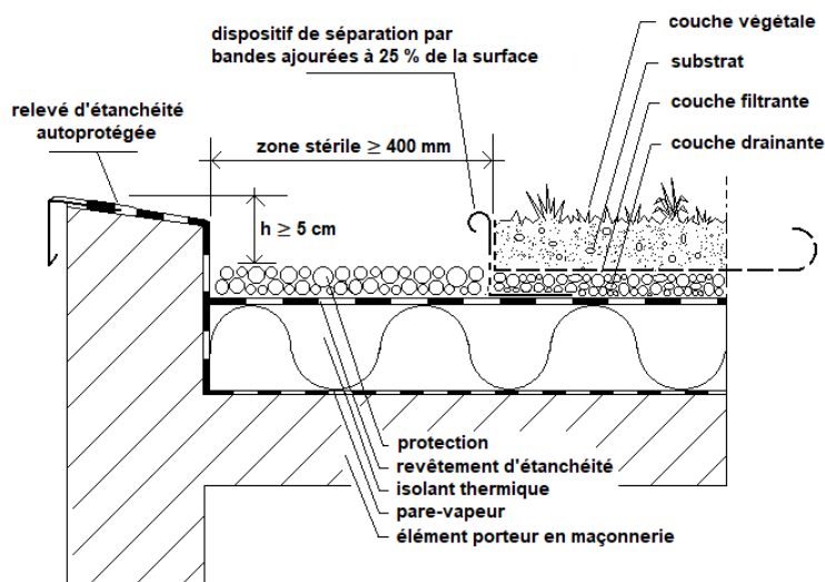
FIGURE 7 CAS PARTICULIER DE L'ACROTÈRE REVÊTU JUSQU'À L'ARÊTE EXTÉRIEURE AVEC ZONE STÉRILE
