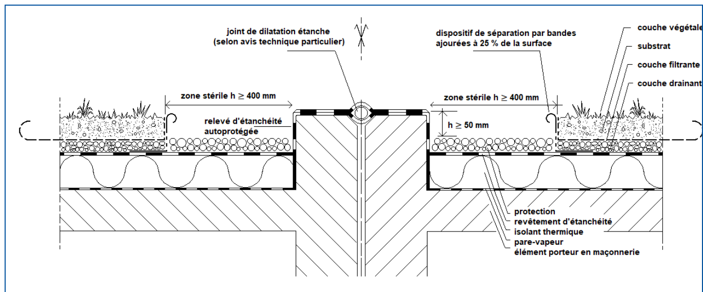
FIGURE 14 JOINT DE DILATATION APPARENT AVEC ZONE STÉRILE
