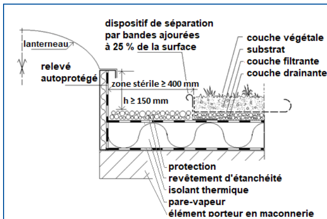
FIGURE 5 RELEVÉ CONTRE COSTIÈRE DE LANTERNEAU AVEC ZONE STÉRILE
