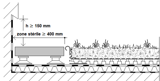
FIGURE 6 RELEVÉ AVEC ZONE STÉRILE TRAITÉE AVEC DALLES SUR PLOTS
